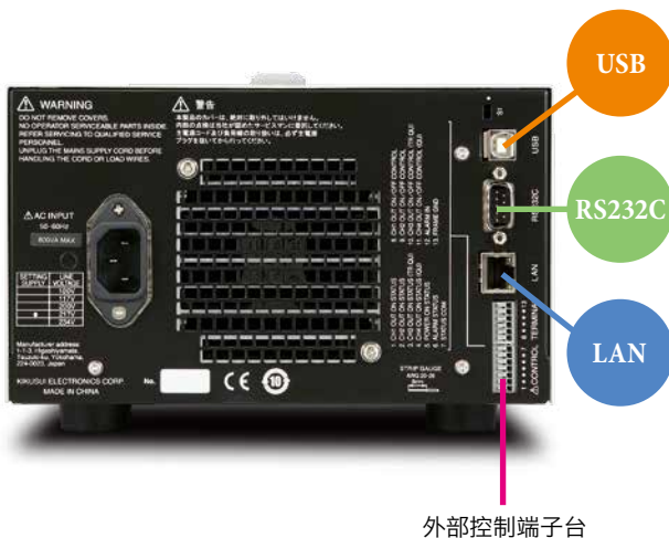
外部控制端子台
